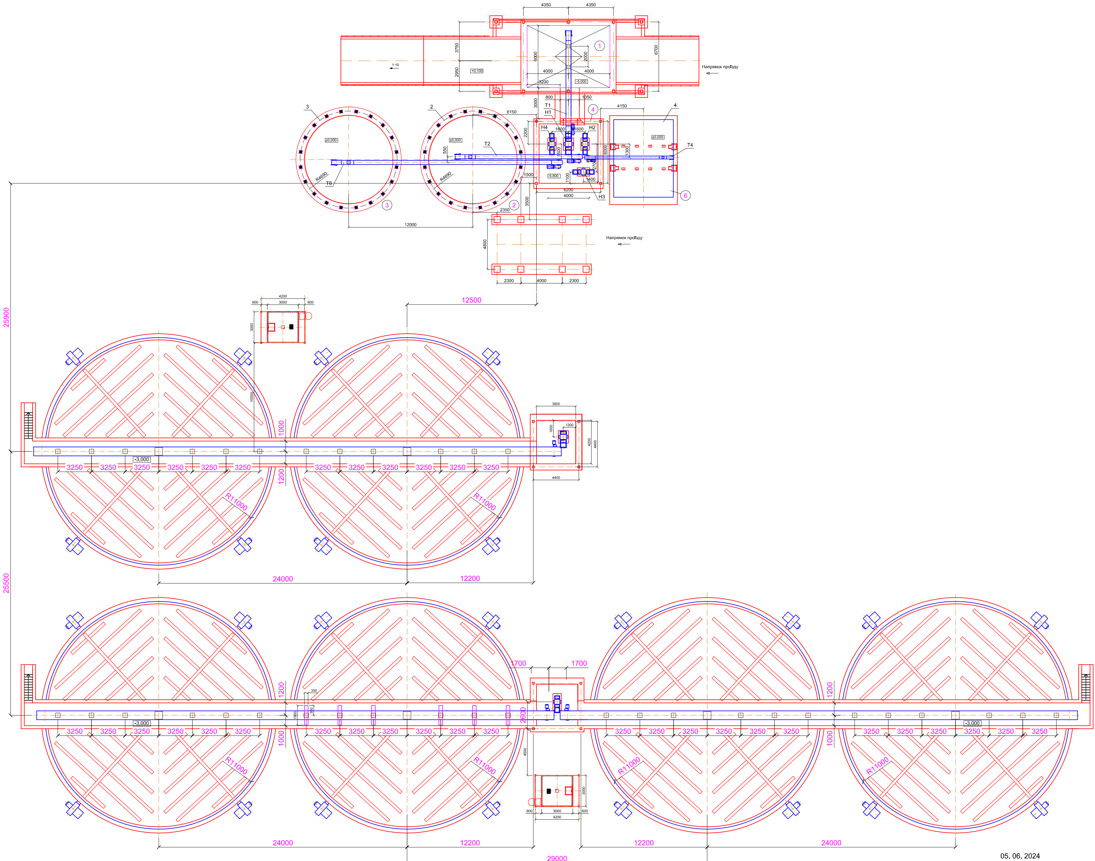
План розміщення технологічного обладнання на відм. \pm 0,000 м
